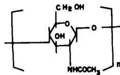
Fig. 1 - Estrutura da quitina
